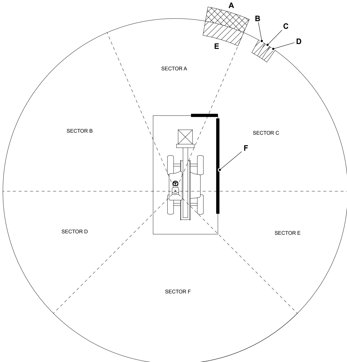
Figura 387. Ocultación de visibilidad en estado de carga de remolque del camión
