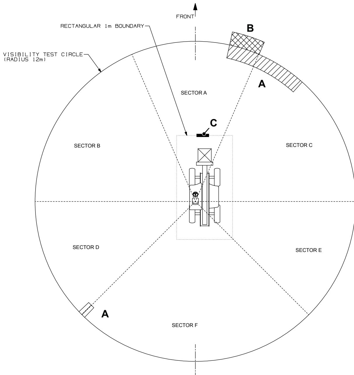
Figura 378. Ocultación de visibilidad en estado de carga de remolque del camión
