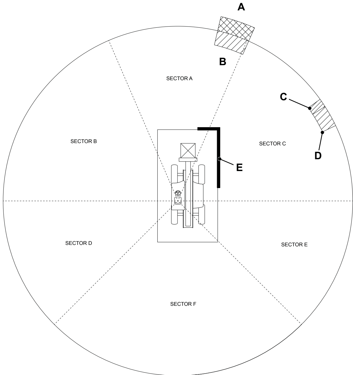
Figura 381. Ocultación de visibilidad en estado de carga de remolque del camión
