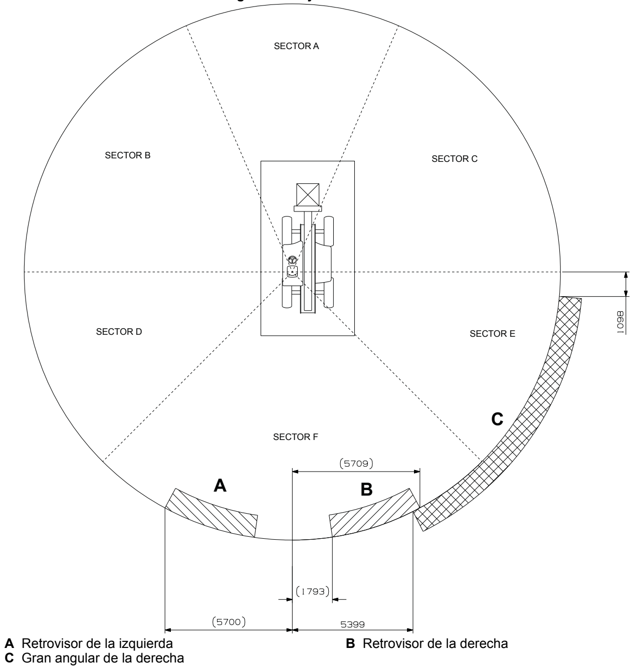
Figura 379. Ajuste del retrovisor
