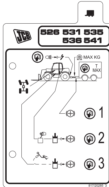
Figura 396. Ejemplo de gráfico de remolcado
