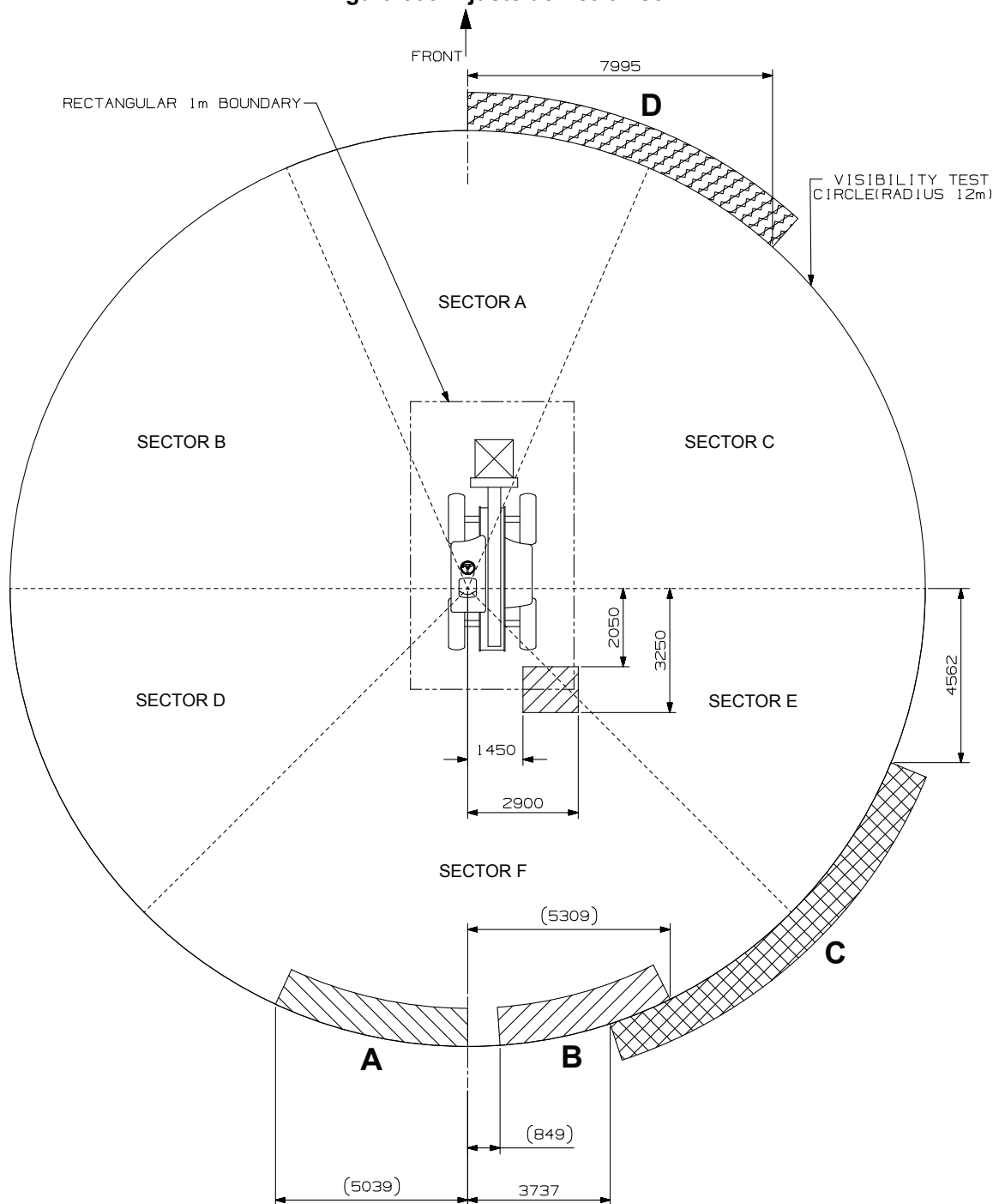
Figura 393. Ajuste del retrovisor
