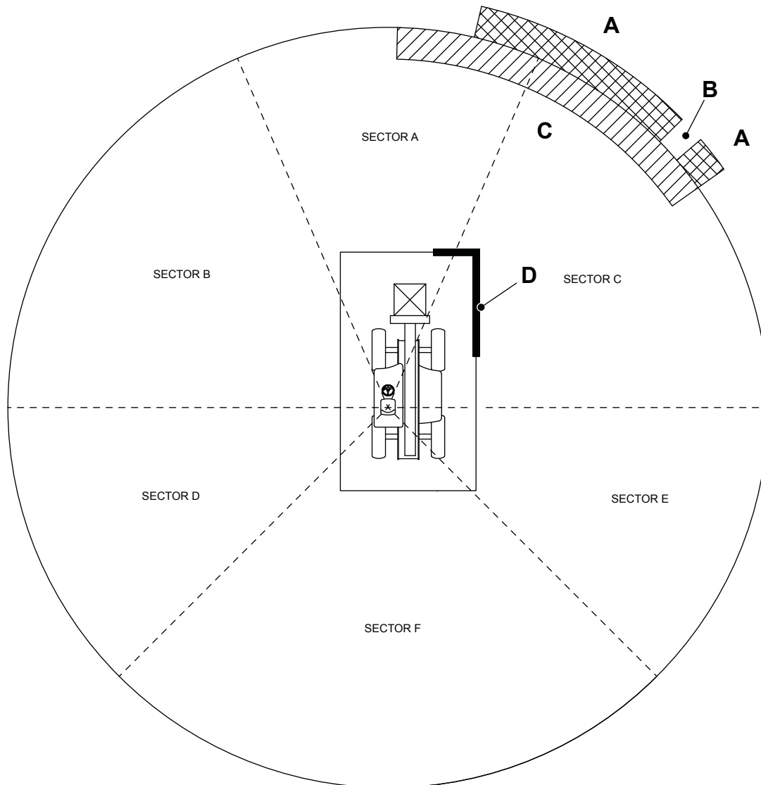
Figura 392. Ocultación de visibilidad en estado de carga de remolque del camión
