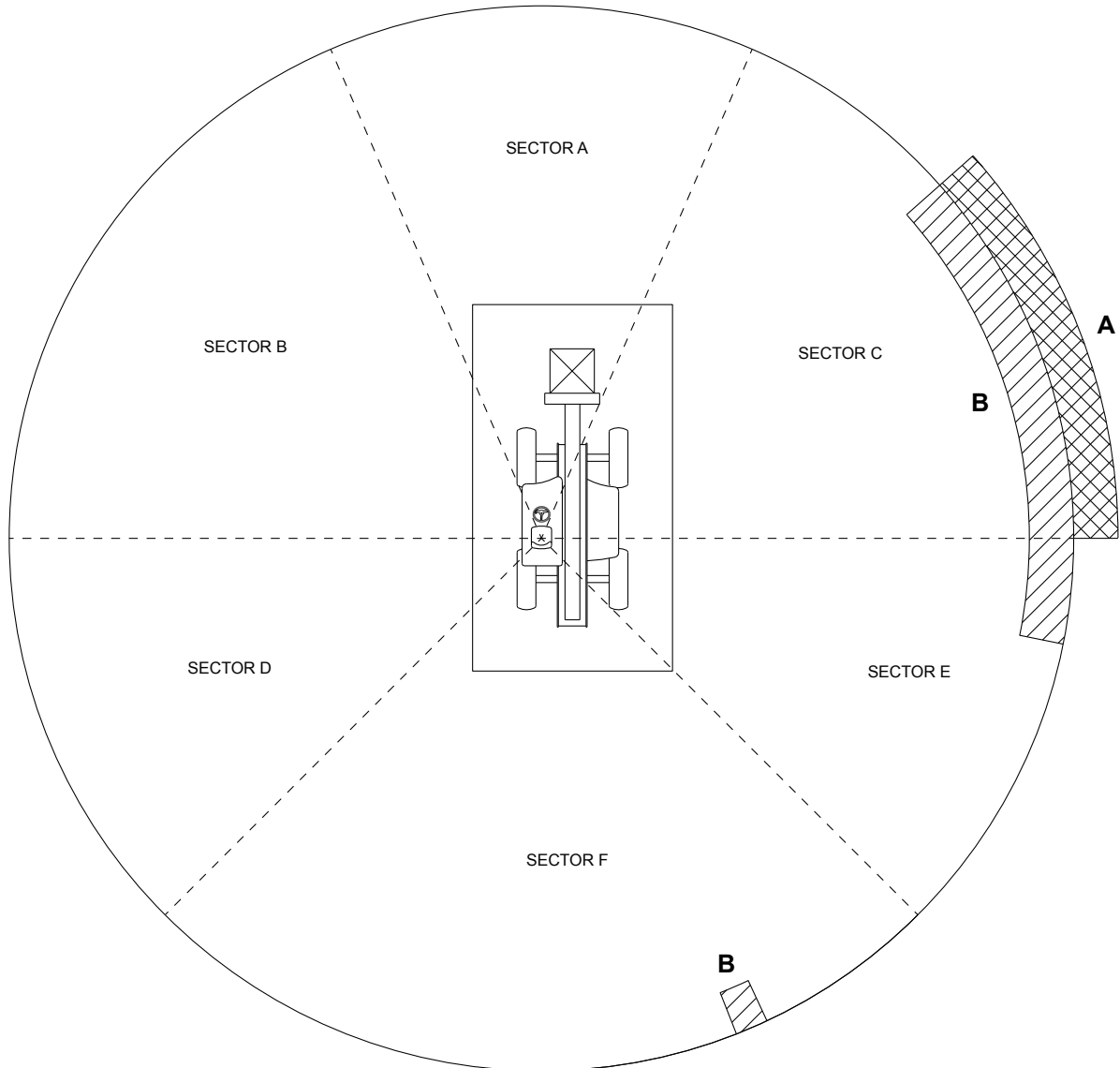
Figura 386. Ocultación de la visibilidad en condición de carga suspendida
