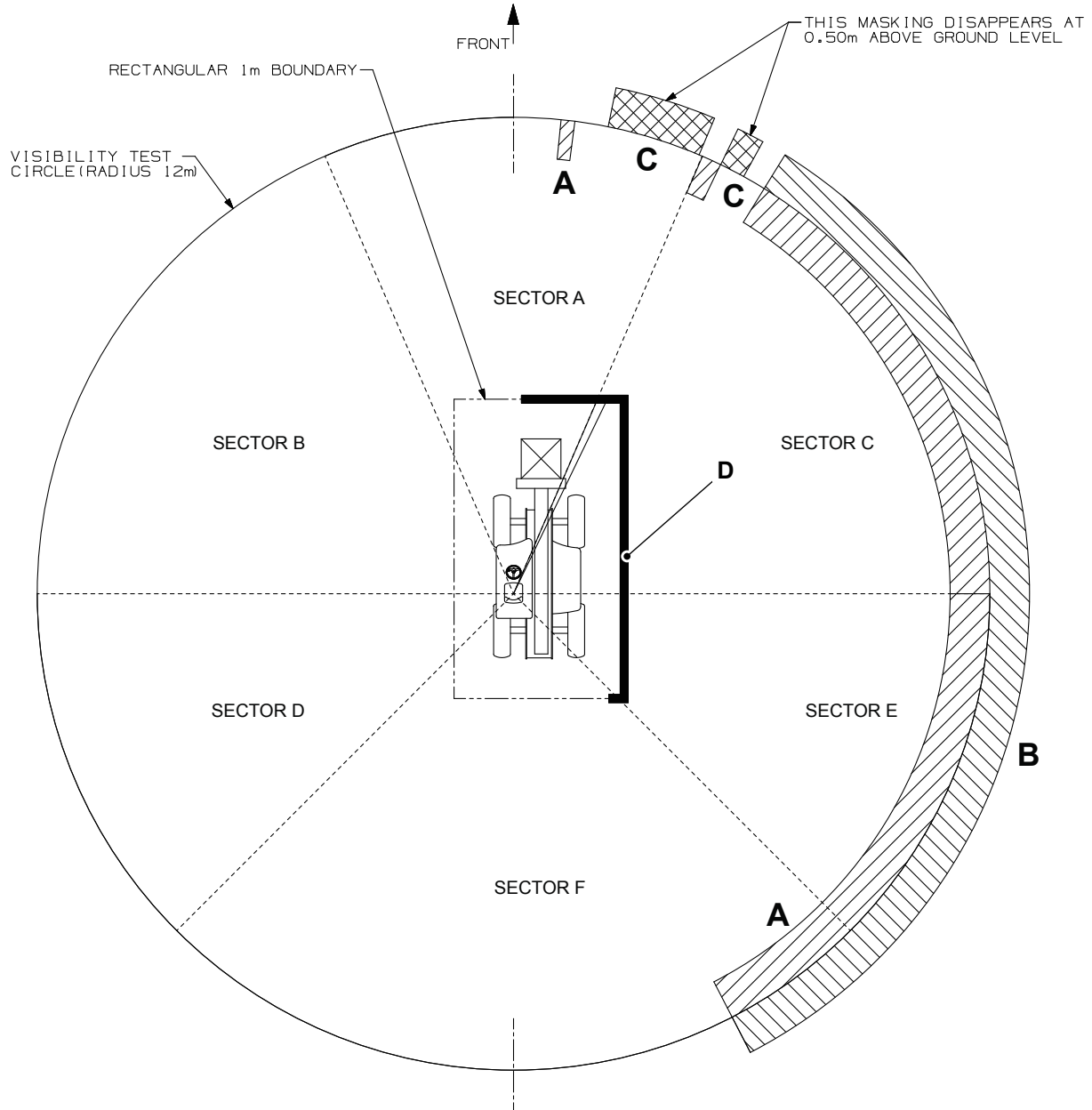
Figura 395. Ocultación de visibilidad en estado de carga de remolque del camión
