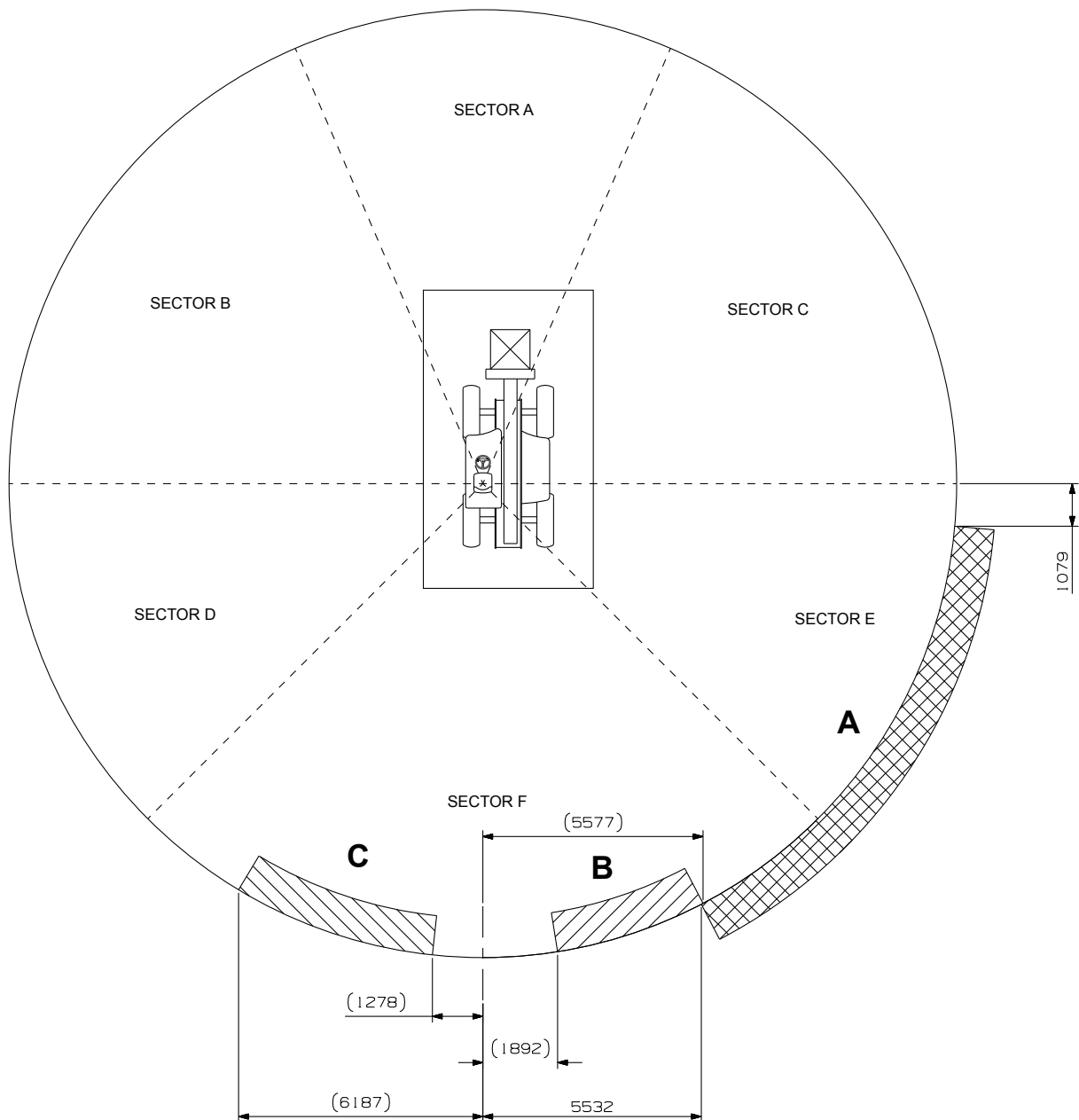
Figura 390. Ajuste del retrovisor
