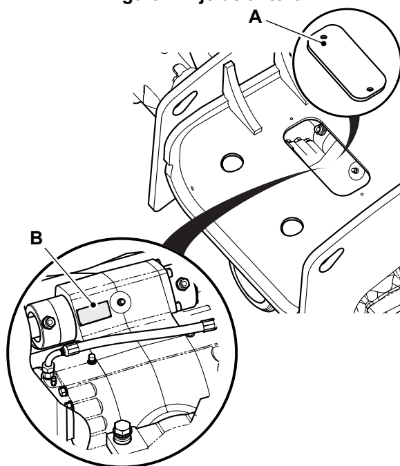
Figura 7. Eje delantero
