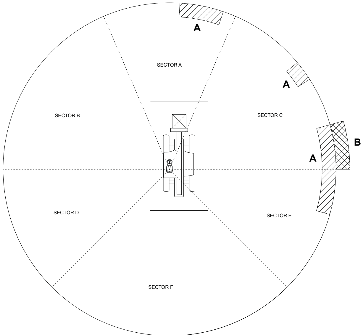
Figura 383. Ocultación de la visibilidad en condición de carga suspendida
