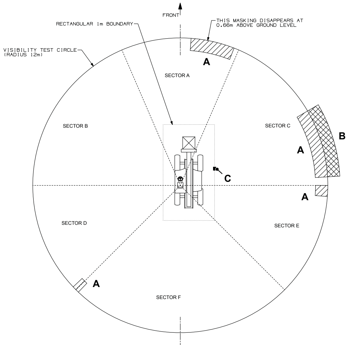
Figura 377. Ocultación de la visibilidad en condición de carga suspendida
