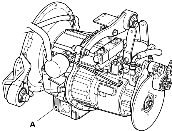
Figura 12. Transmisión Syncro Shuttle
