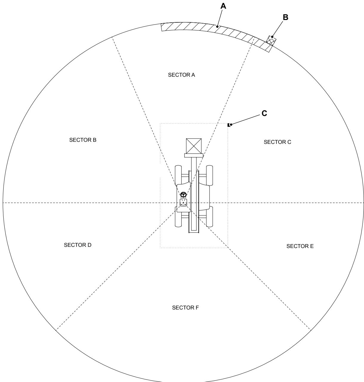
Figura 388. Ocultación de visibilidad - pala para cereales
