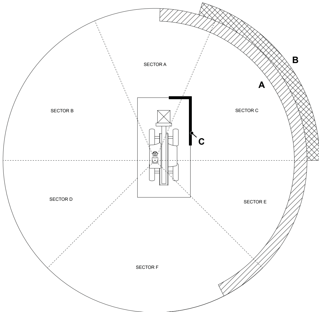
Figura 384. Ocultación de visibilidad en estado de carga de remolque del camión
