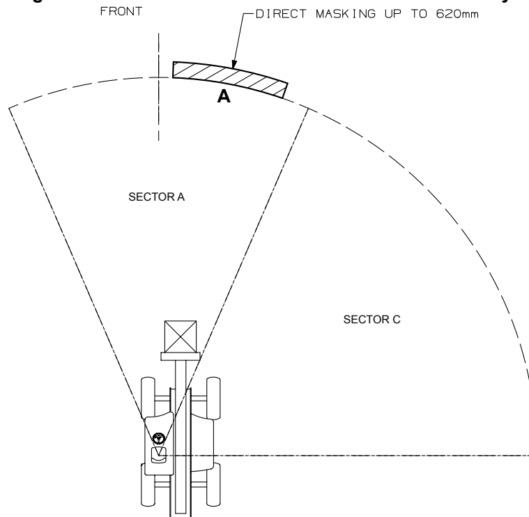
Figura 389. Ocultación de visibilidad en los sectores A y C
