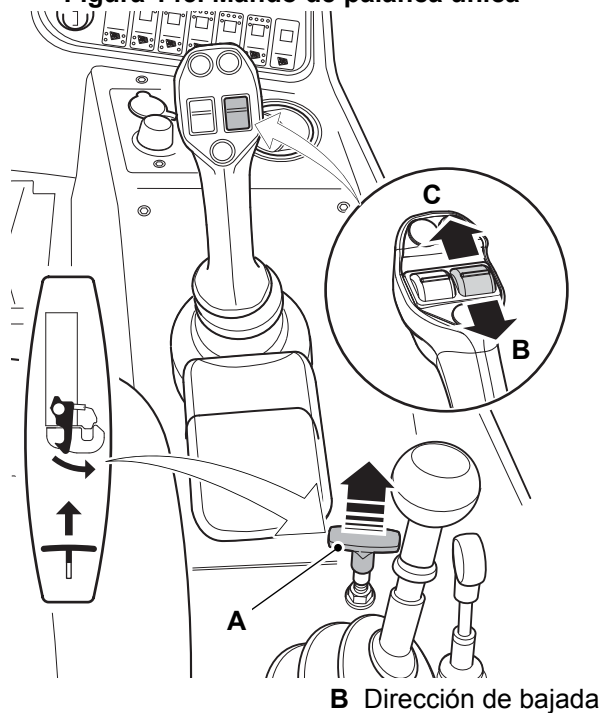
Figura 145. Mando de palanca única
