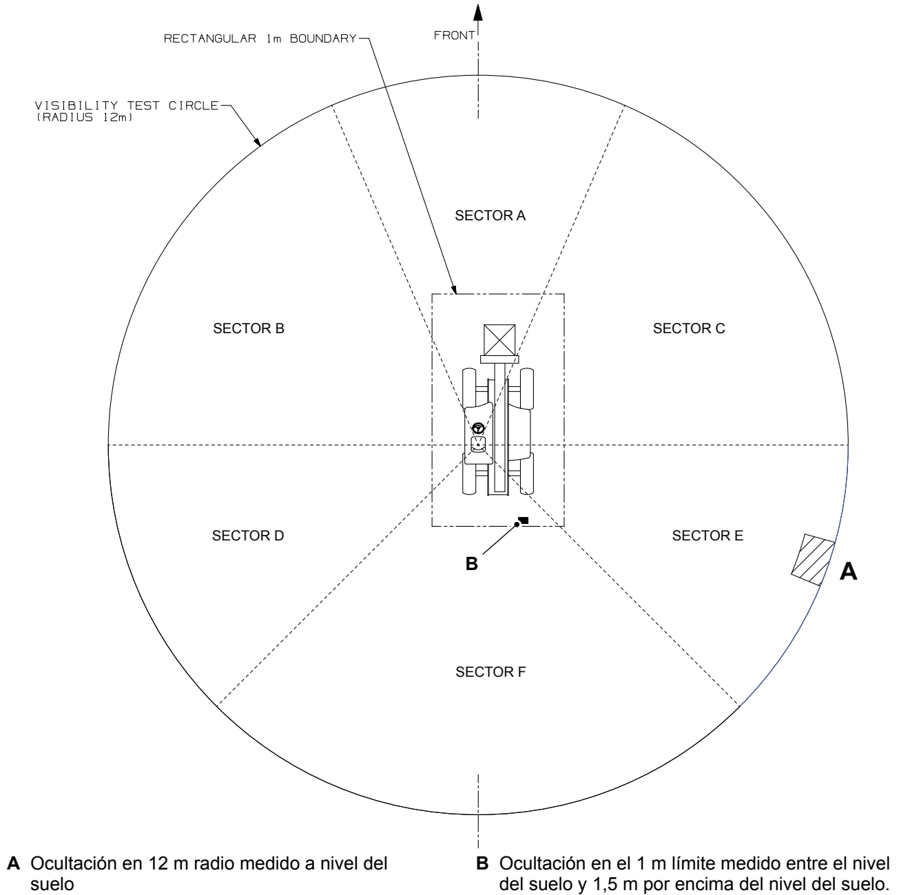
Figura 394. Ocultación de la visibilidad en condición de carga suspendida
