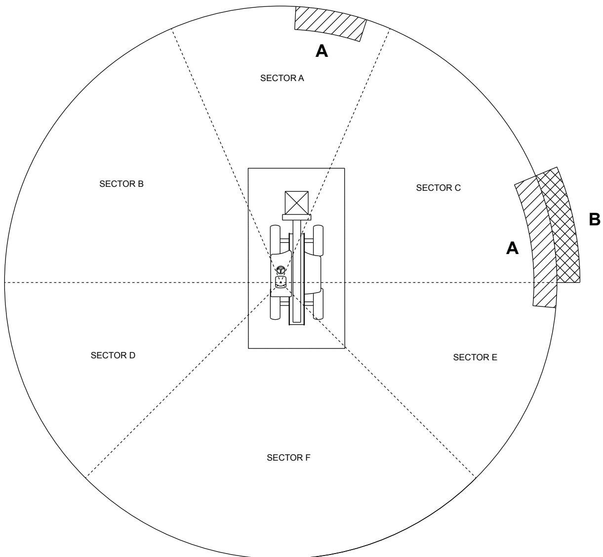
Figura 380. Ocultación de la visibilidad en condición de carga suspendida
