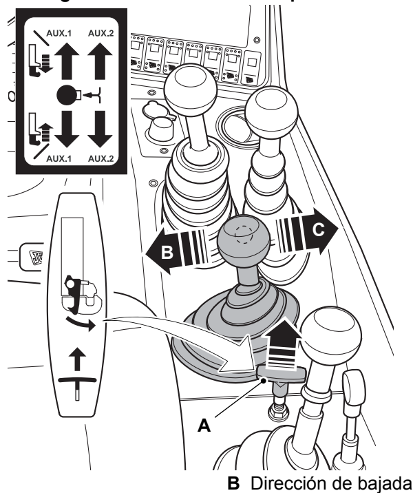
Figura 144. Mando de doble palanca
