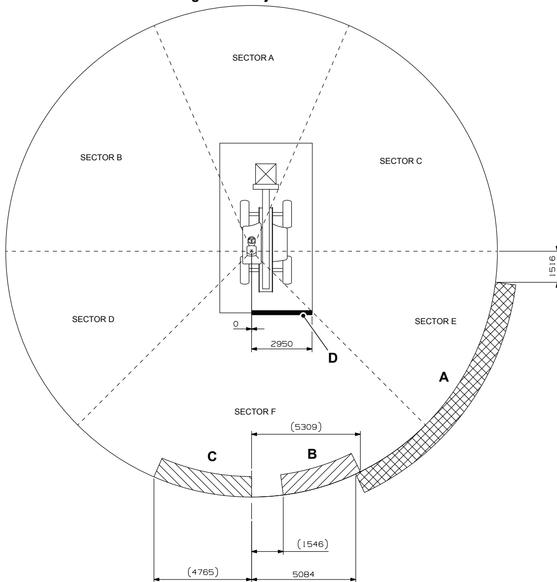
Figura 385. Ajuste del retrovisor
